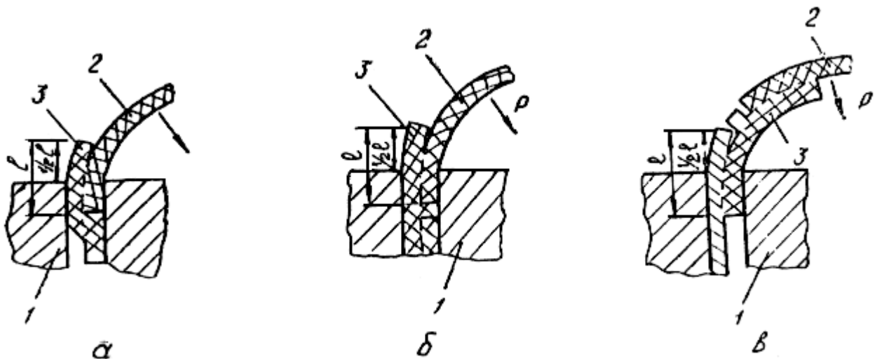
Рис. 16. Схема испытания сварных соединений на отдир: а - раструбное соединение; б, в - раструбно-стыковое соединение; 1 - зажимное устройство;
