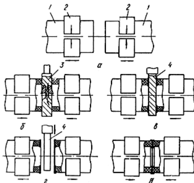
Рис.6. Схема контактной сварки встык:
