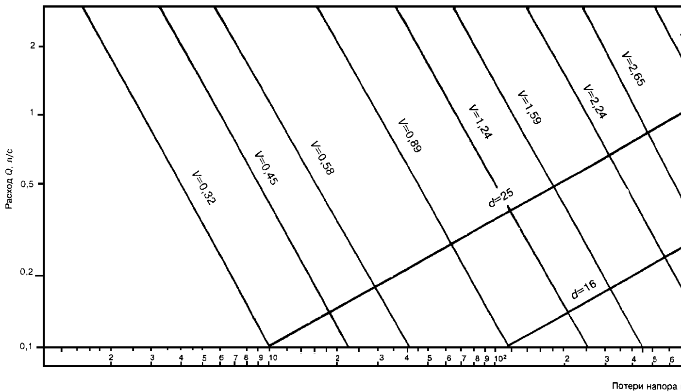
Рисунок А.1 - Номограмма для приближенного гидравлического расчета водопровода холодной воды из металлополимерных труб по ТУ 2248-001-07629379-96
