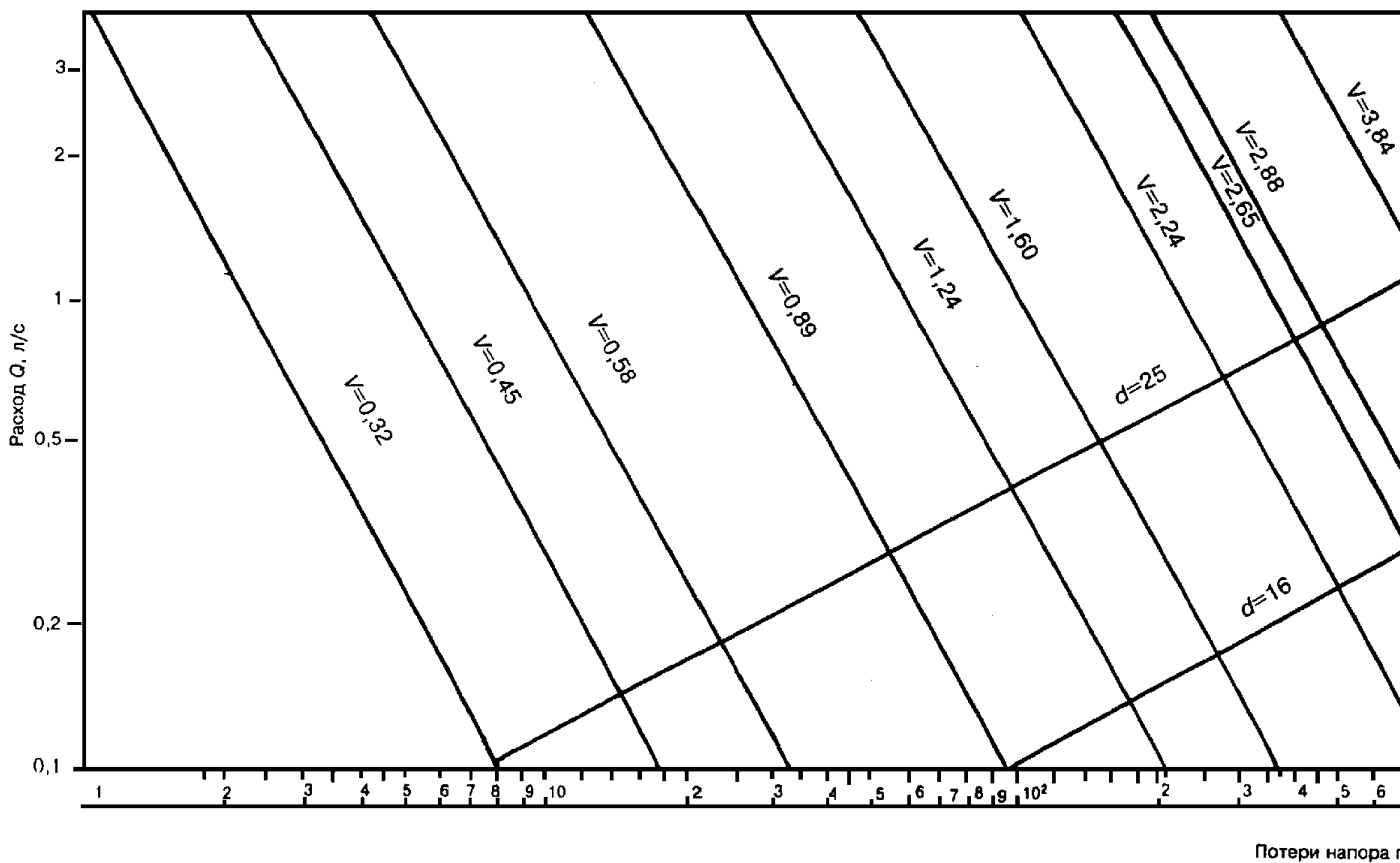
Рисунок А.2 - Номограмма для приближенного гидравлического расчета водопровода горячей воды из металлополимерных труб по ТУ 2248-004-07629379-97
